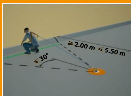
individueel ankerpunt
